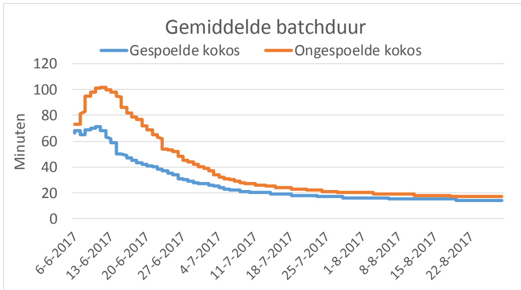
Figuur 5. Gemiddelde behandelduur van een batch water, waarbij 1 minuut voorbehandeltijd, en 5 minuten nabehandeltijd standaard zijn ingesteld in onze emissieloze teelt. Streefwaarde voor ontsmetting is een redoxwaarde van 800 mV.
