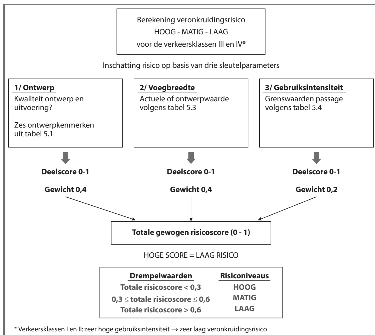
Figuur 5.2 Berekening van het veronkruidingsrisico (enkel voor de verkeersklassen III en IV)
