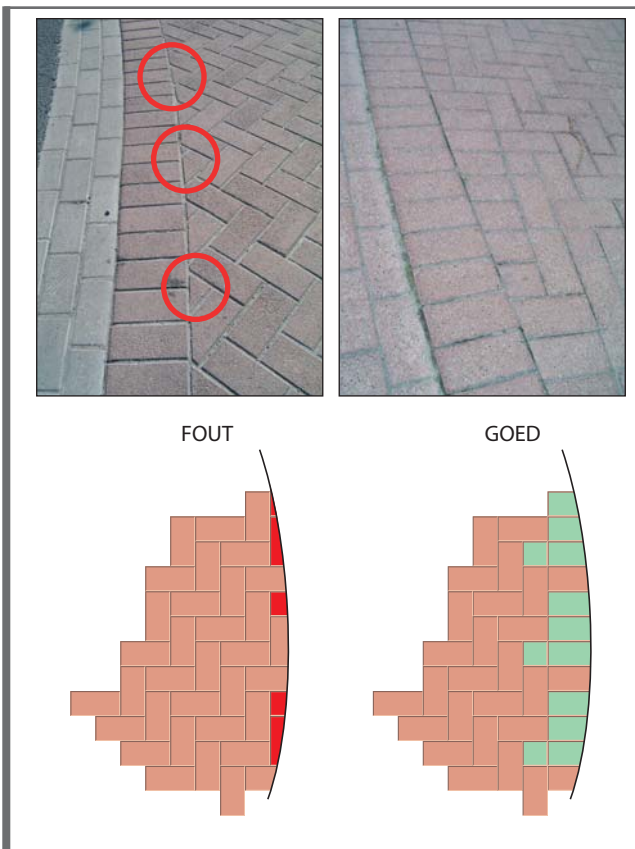
Figuur 3.4 Foutieve en goede randafwerking in een bocht
