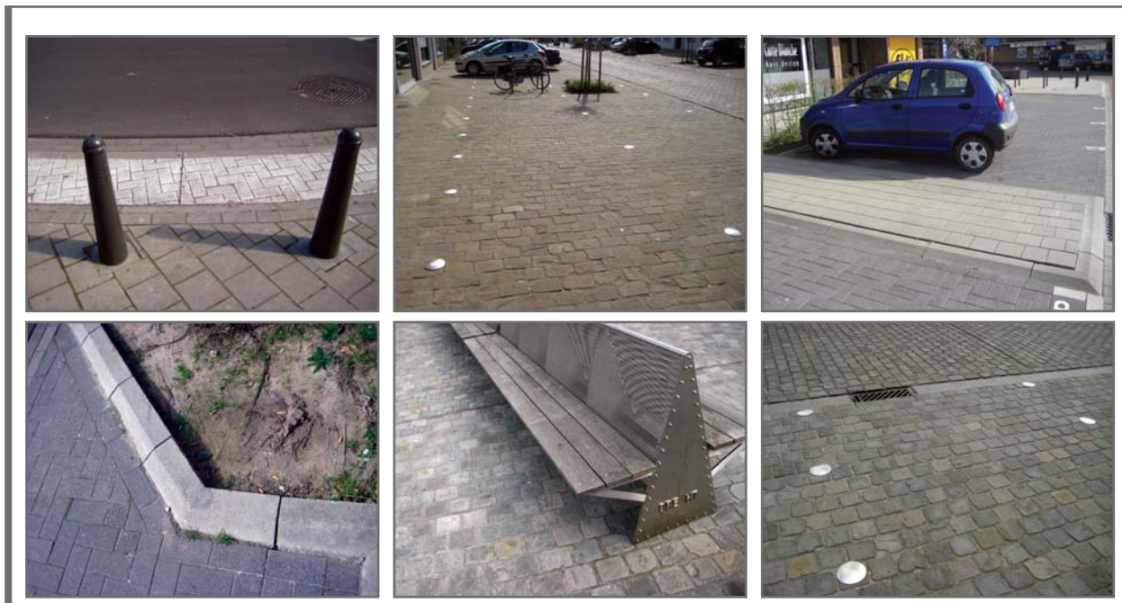
Figuur 3.20 Aandacht in het ontwerp voor machinaal onderhoud bij toekomstig curatief onkruidbeheer: voldoende afstand tussen obstakels, verwijderbare obstakels, vloeiende overgangen tussen de rijbaan en het fiets- of voetpad, kantstenen met afgeschuinde hoeken, straatgoot tussen de parkeervoorziening en de rijbaan
