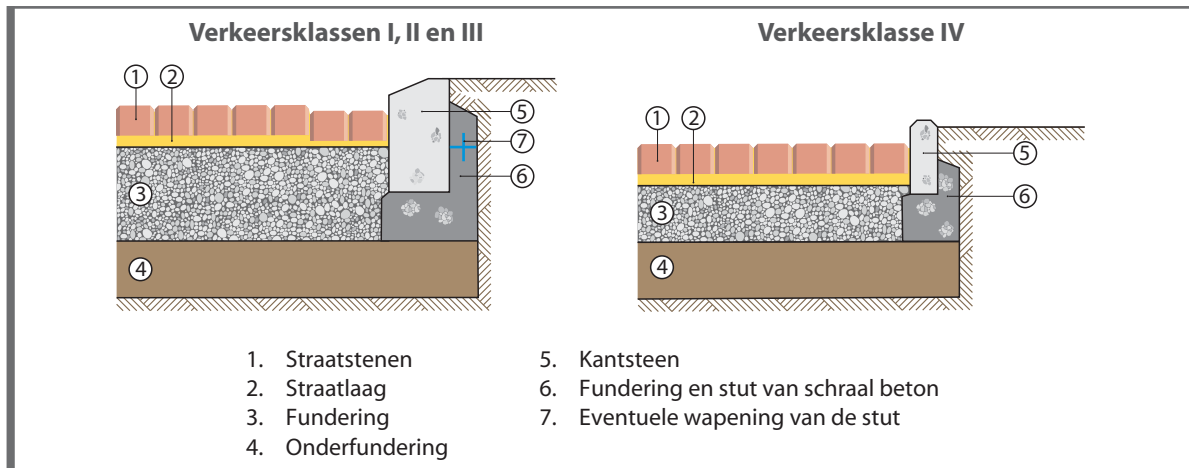
Figuur 3.12 Kantopsluiting naargelang van de verkeersklasse
