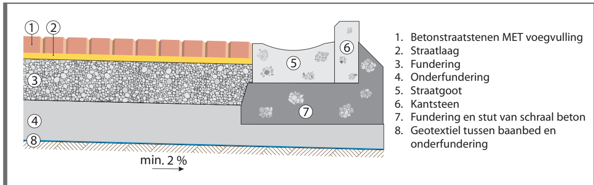
Figuur 1.1 Standaardopbouw van steenbestrating
