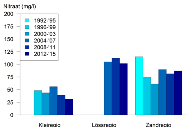
Figuur 10. Gemiddelde nitraatconcentratie (als \text{NO}_3 in mg/l) in het water dat uitspoelt uit de wortelzone van akkerbouwbedrijven in LMM per regio en periode (Fraters et al., 2016).
